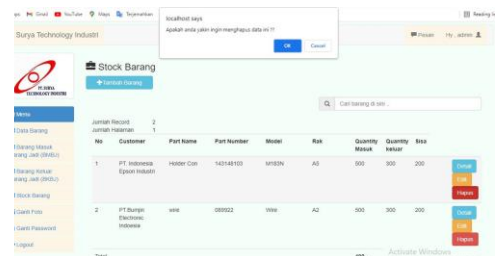
Gambar 4.6 Tampilan hapus
