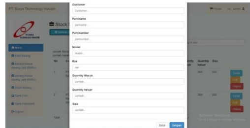
Gambar 4.4 Tampilan Input
