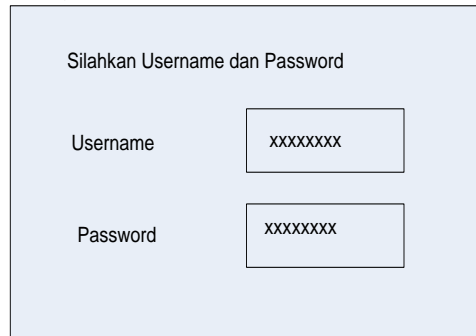
Gambar 4 Login
