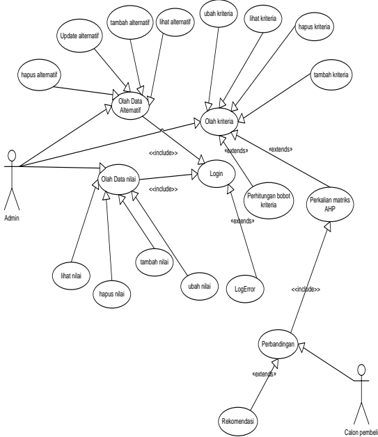
Gambar 7 Use Case Sistem Pengambilan Keputusan Bibit Jagung
