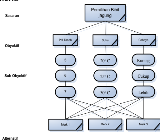
Gambar 5 Bagan Kriteria
